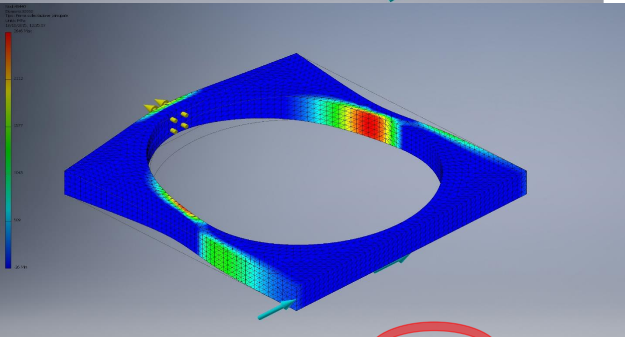
Prima sollecitazione: \sigma_{\text{MAX}} = 2646 \text{ MPa}
