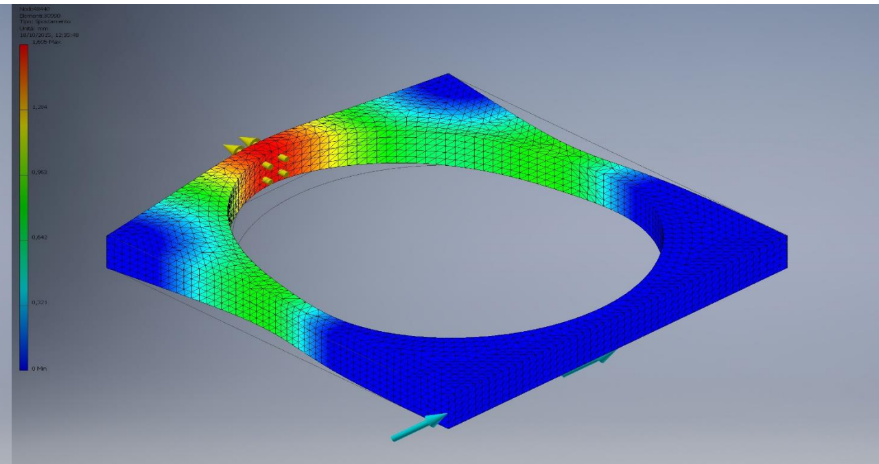
Spostamento: dL_{\text{MAX}} = 1,605 \text{ mm}
